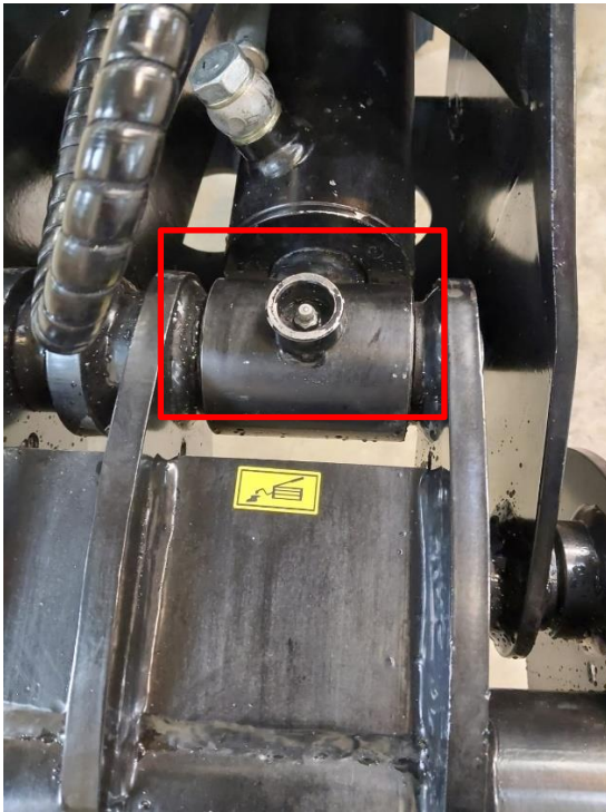
Abbildung 9: Schmierstellen Zylinder
