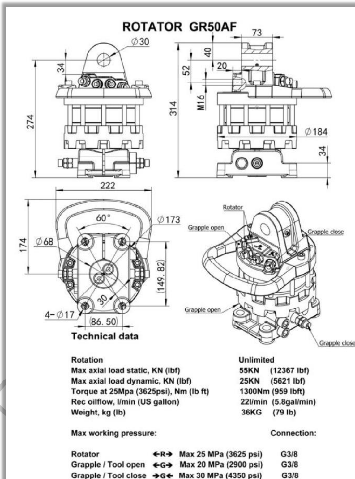
Abbildung 3: Datenblatt Rotator GR50AF
