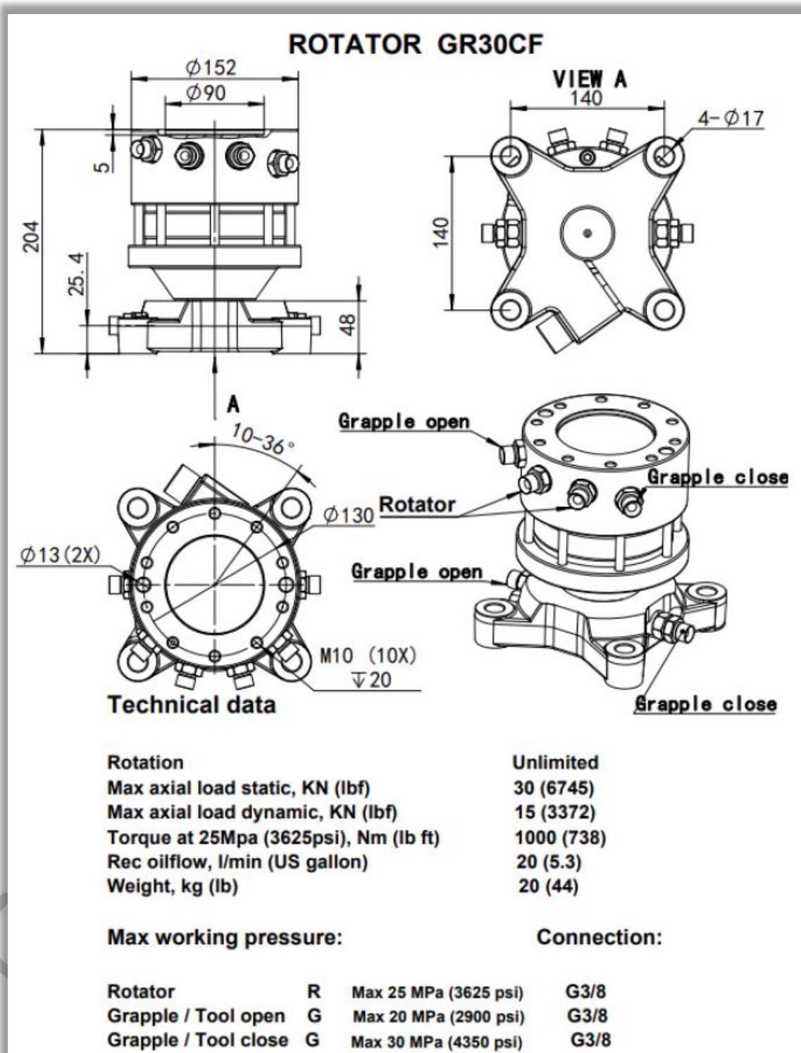
Abbildung 4: Datenblatt Rotator GR30CF
