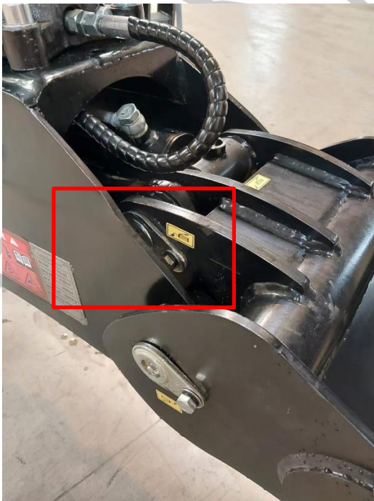
Abbildung 10: Schmierstellen Gelenk
