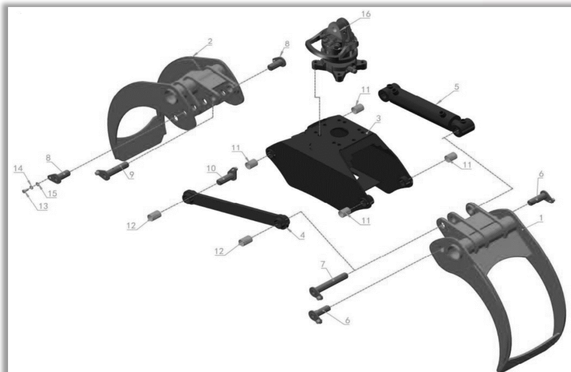
Abbildung 11: Ersatzteilliste Forstgreifer
