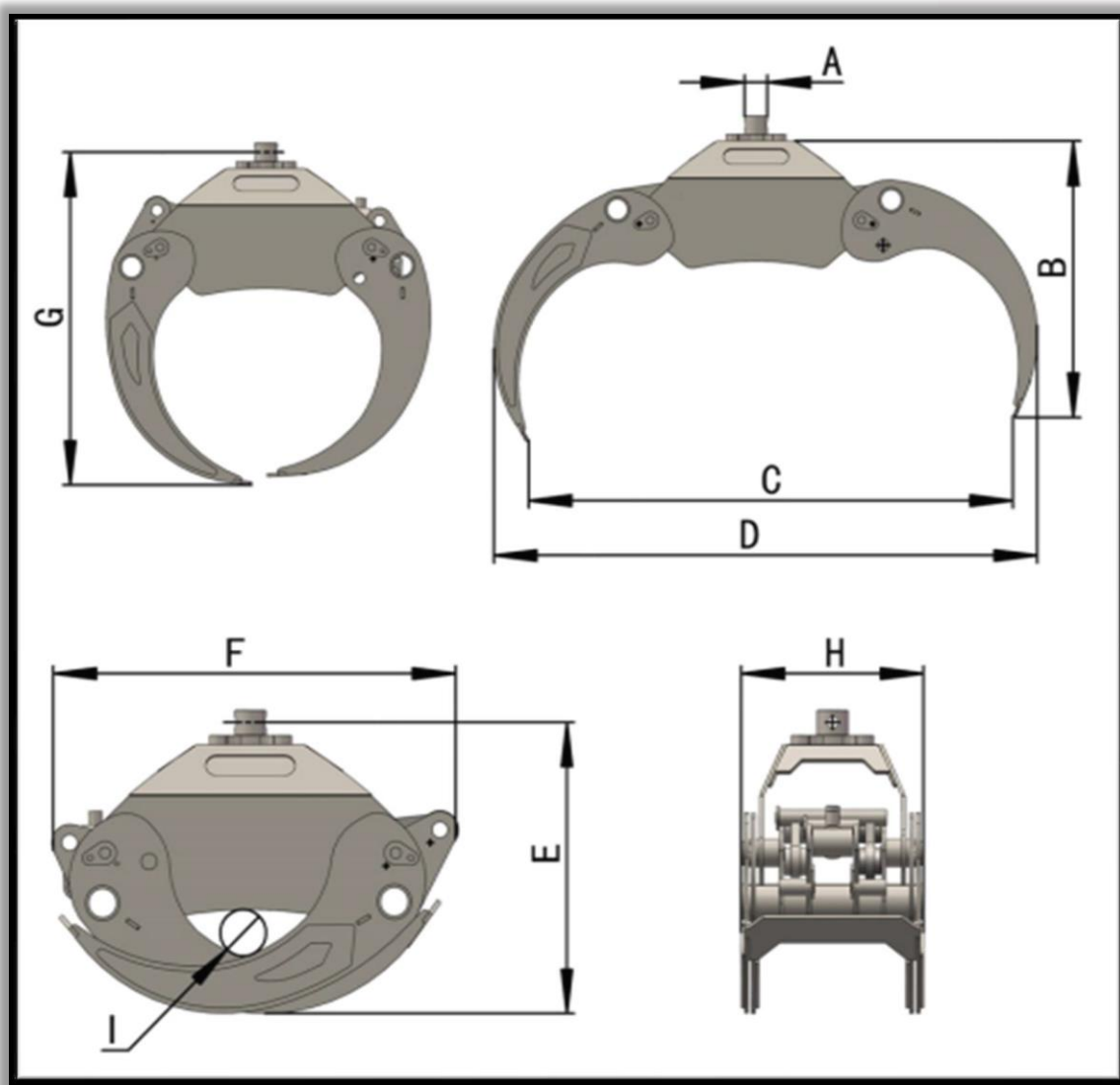
Abbildung 1: Abmessungen Forstgreifer
