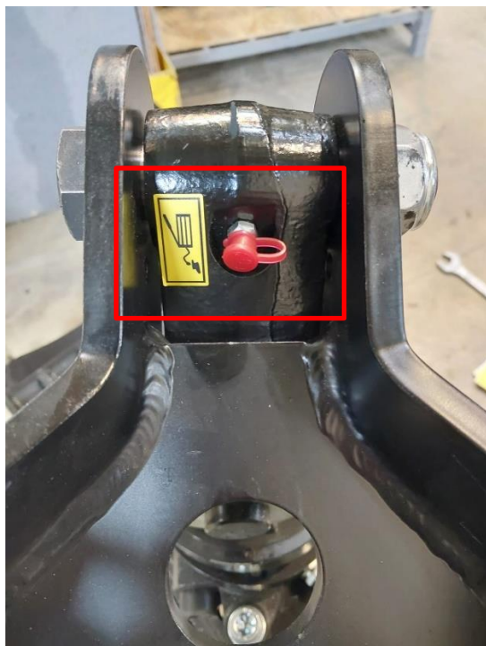
Abbildung 7: Schmierstellen Pendelgelenk
